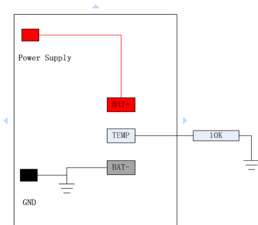
图 3-2 NTC 夹具接线方法
