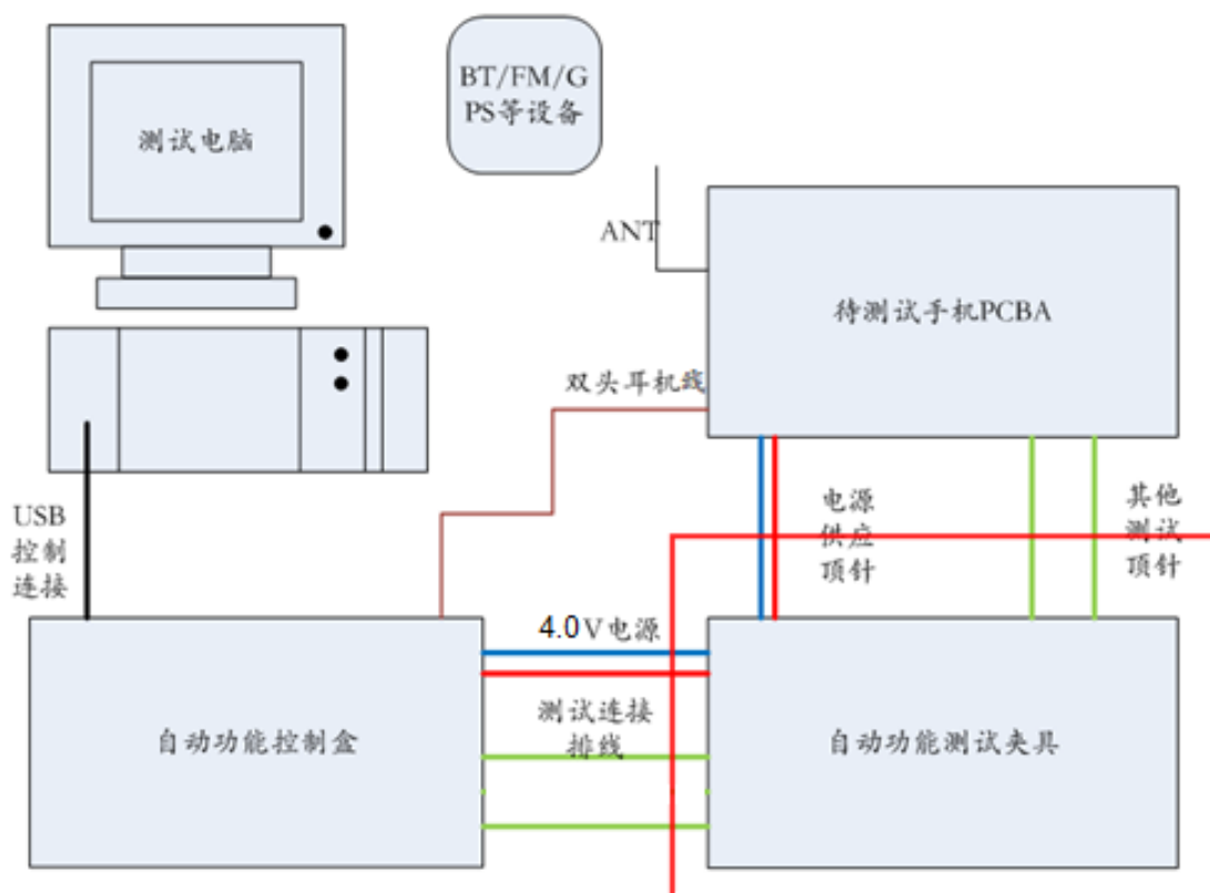
图 1-1 自动功能测试模块连接示意图
